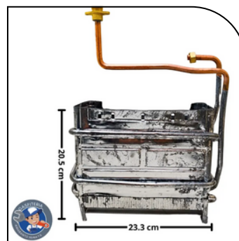
SERPENTIN 7-8L MASTER (MULTIVALVULA)
