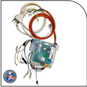
MODULO DE ENCENDIDO T.F JUNKERS WR 11 -13 -16
